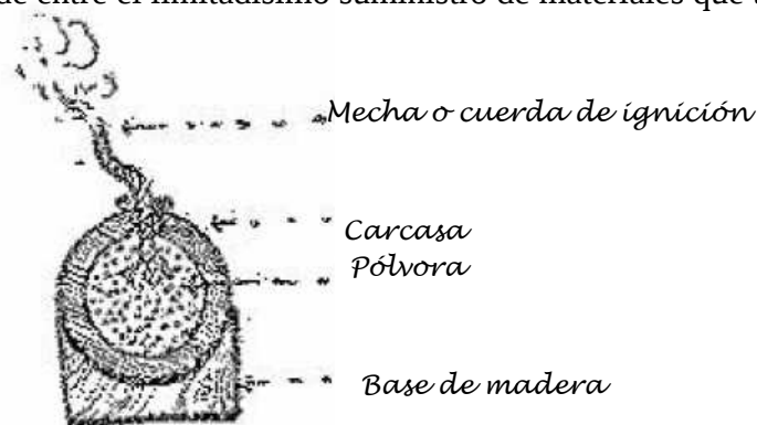
SECCIÓN DE UN OBÚS
